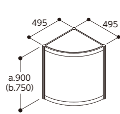
5 1/4R展示台(a.b)
