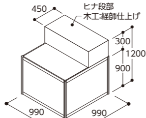
3 システムひな段
