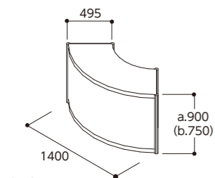
7 R展示台(a.b)
